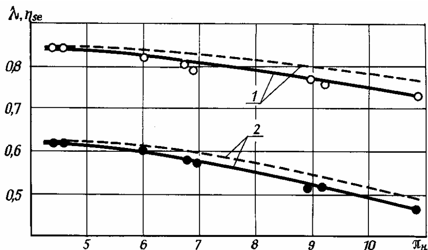
Рис. 2. Зависимость расчетных и экспериментальных величин коэффициентов подачи \lambda (1) и изэнтропных эффективных КПД \eta_{se} (2) холодильного ВКМ от степени сжатия \pi_k : ----- эксперимент (по данным работы [3]); - - - - расчет
